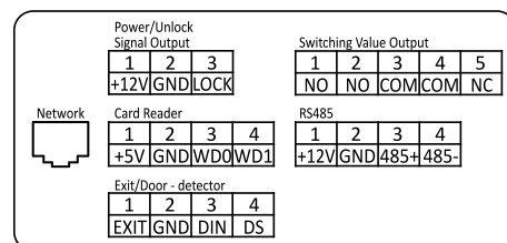
Terminal przyłączeniowy
